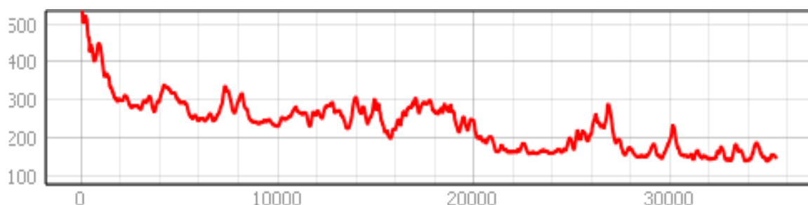
Gráfico 1 – Perfil topográfico do rio principal do Rio Gandu.
