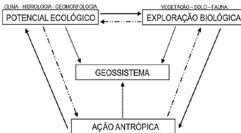
Figura 3 – Fluxograma teórico do Geossistema para Bertrand
