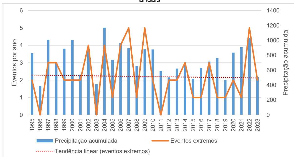
Gráfico 5 - Relação entre pluviometria acumulada e a quantidade de eventos extremos anuais
